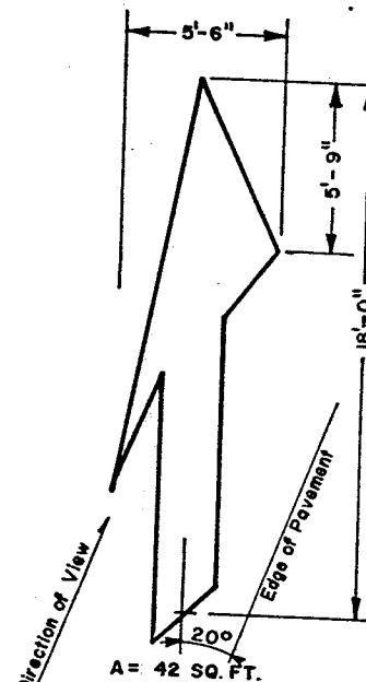
TYPE VI ARROW
