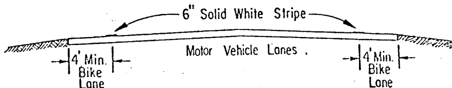
(D) TYPICAL ROADWAY IN OUTLYING AREAS
